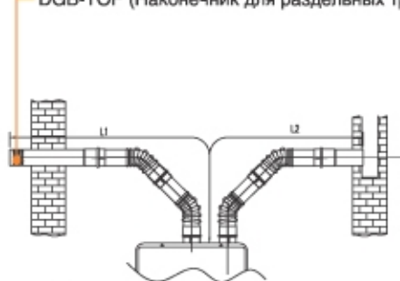
DGB-TOP (Наконечник для раздельных труб)
