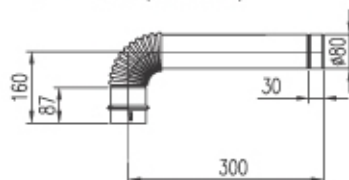
DGB-EL90 (Угол 90°)
