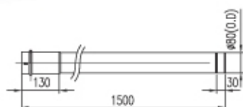
DGB-S1500 (Труба прямая 1500 мм.)
