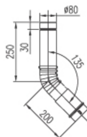
DGB-EL45 (Угол 45°)
